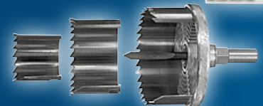
8dielna sada dierových píľ Ø 25/32/38/44/51/57/63/68 mm
